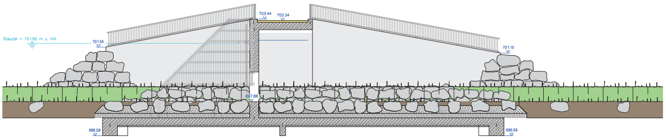
Schnitt A-A mit Gestaltung
